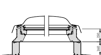
RWA-Flachdach-Fenster CSP (15-cm-Rahmenhöhe) mit fix montiertem, 16 cm hohem Aufsetzkranz (Gesamthöhe 31 cm)
